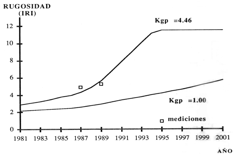
Fig.4 Ajuste al modelo de irregularidad superficial
