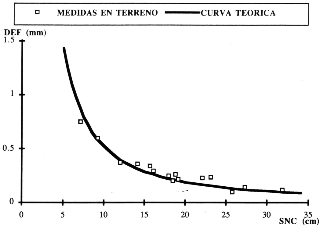
Fig.5 Relación entre la deflexión con viga Benkelman y el número estructural corregido
