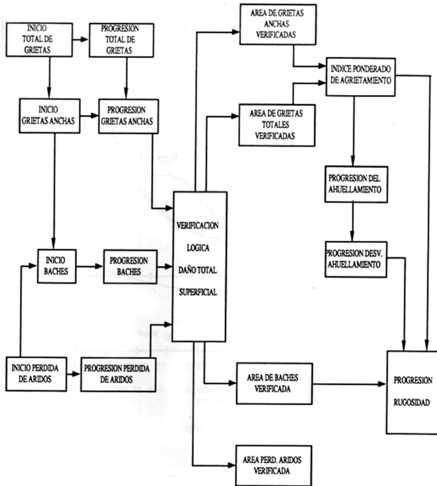
Fig.3 Relación entre los modelos de deterioro del HDM-III
