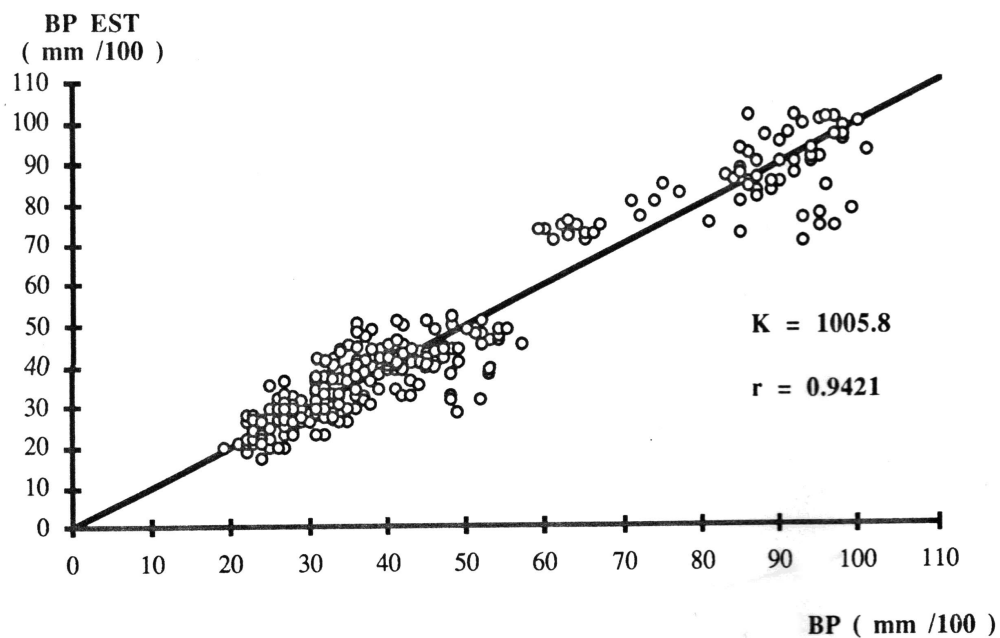
Fig.6 Comparación entre las deflexiones medidas con base de referencia profunda y las estimadas mediante corrección geométrica del deflectómetro transitivo
