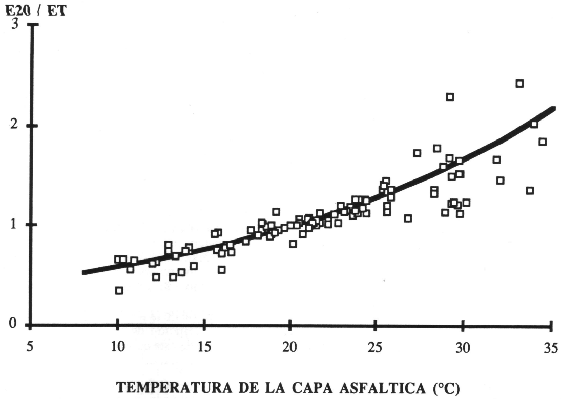
Fig.7 Variación del módulo de elasticidad con la temperatura
